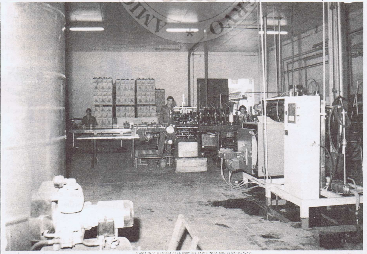
PLANTA EMBOTELLADORA DE LA COOP. DEL CAMPO "NTRA. SRA. DE MANJAYACAS"
